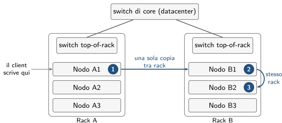
Figura 1.4. Posizionamento di default delle repliche in HDFS, con fattore 3. Una sola copia attraversa la rete tra i rack; se si guasta un rack intero, nell'altro resta almeno una replica.
